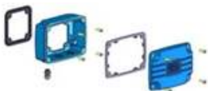
Caixa de ligação (Carcaça 71 a 200)
