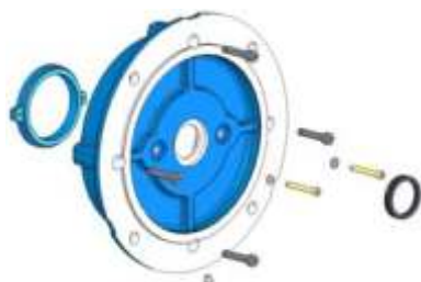
Flange para motoredutores (Carcaça 63 a 180)
